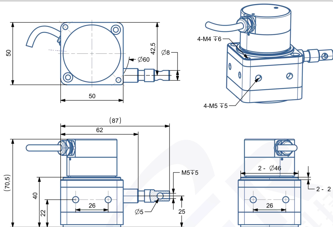
IP68/防爆款 BRT38 系列 0.3/0.5/1 米拉绳位移传感器安装尺寸图
