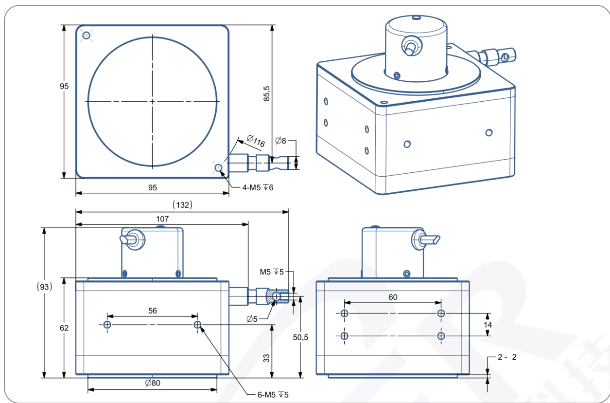
IP54 BRT38 系列 6/7 米拉绳位移传感器安装尺寸图
