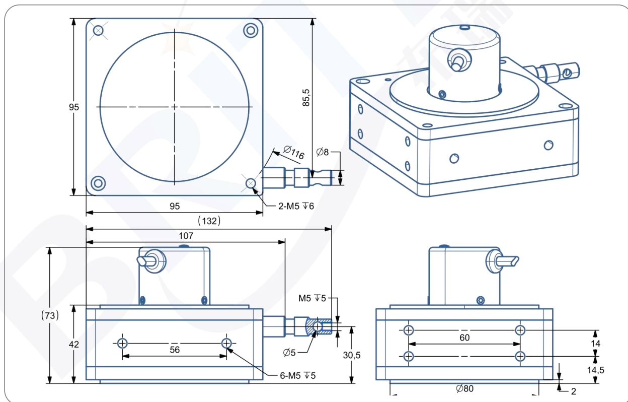
IP54 BRT38 系列 4/5 米拉绳位移传感器安装尺寸图
