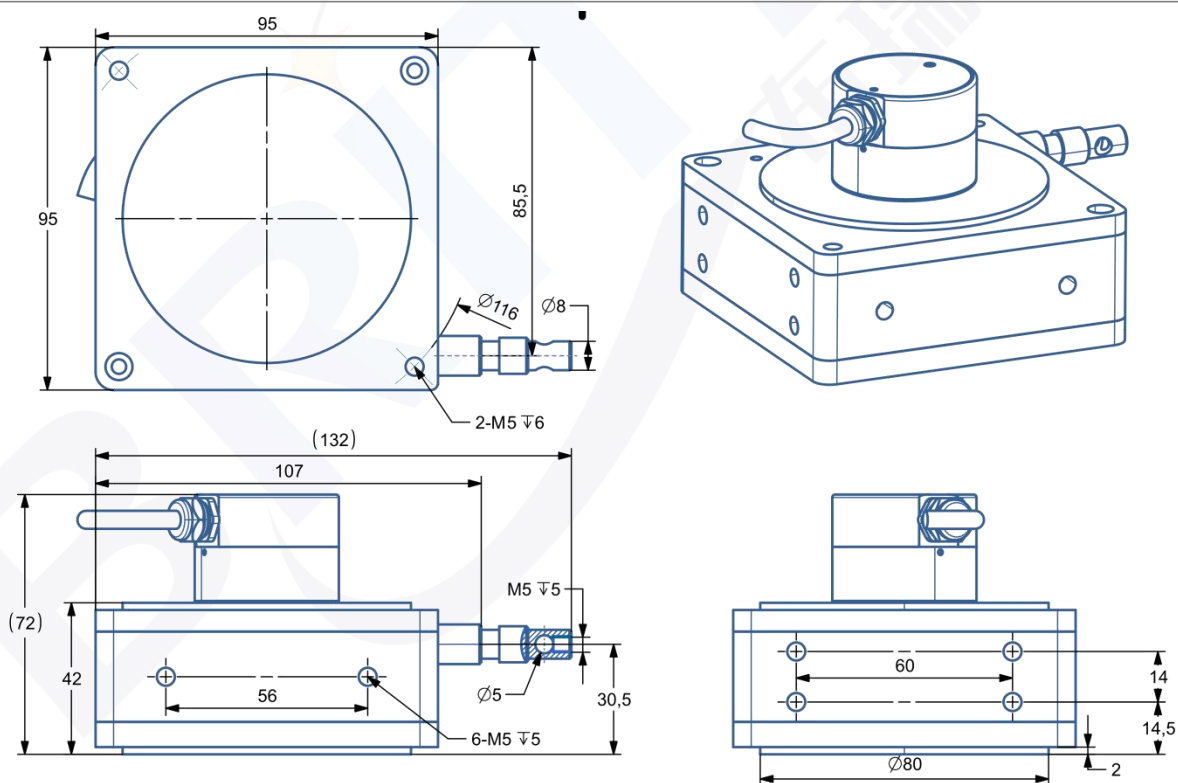
IP68/防爆款 BRT38 系列 4/5 米拉绳位移传感器安装尺寸图
