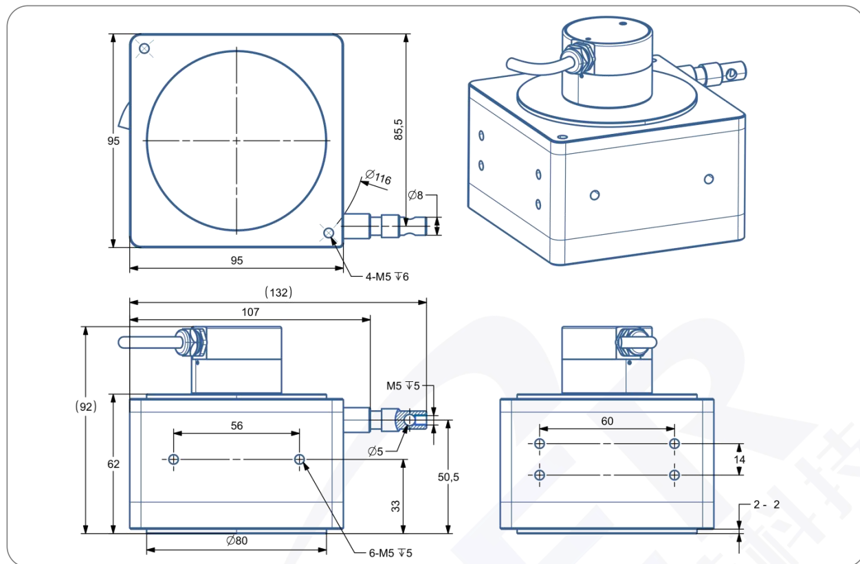
IP68/防爆款 BRT38 系列 6/7 米拉绳位移传感器安装尺寸图
