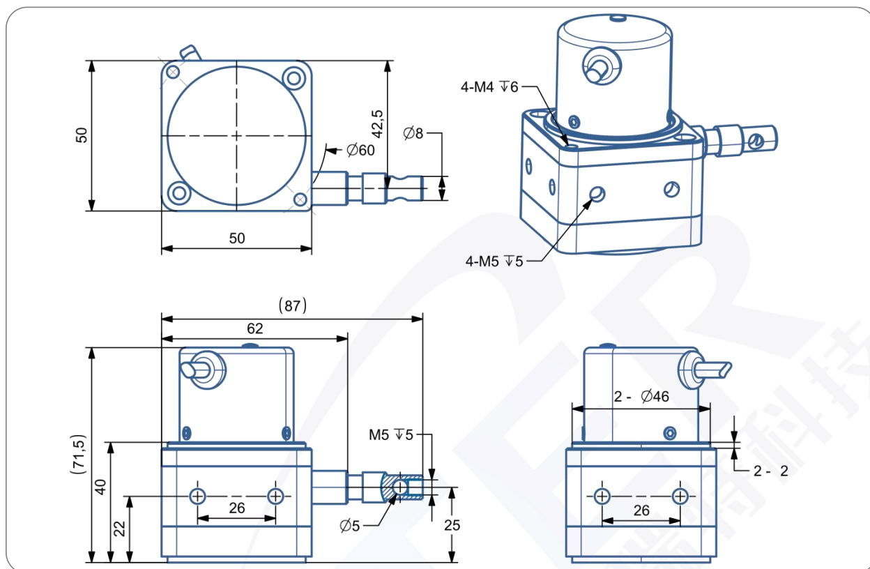
IP54 BRT38 系列 0.3/0.5/1 米拉绳位移传感器安装尺寸图
