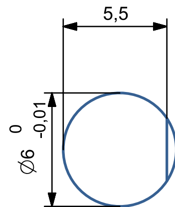
D 字型轴尺寸 比例 5 : 1
