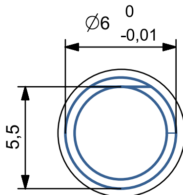
D 字型轴尺寸 比例 5 : 1
