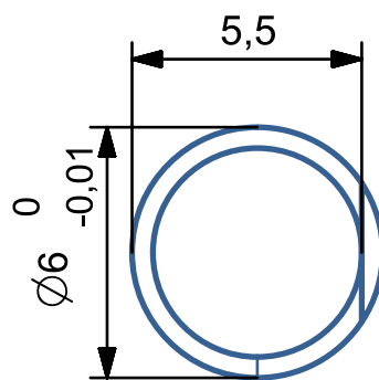
D 字型轴尺寸 比例 5 : 1
