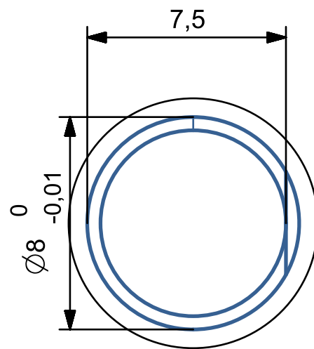
D 字型轴尺寸 比例 5 : 1
