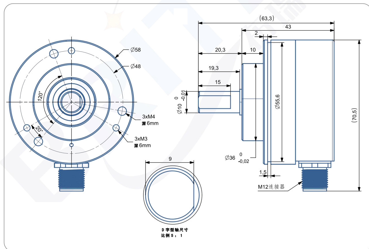
尺寸型号图 12: 输出轴 10mm IP54/IP68/防爆
