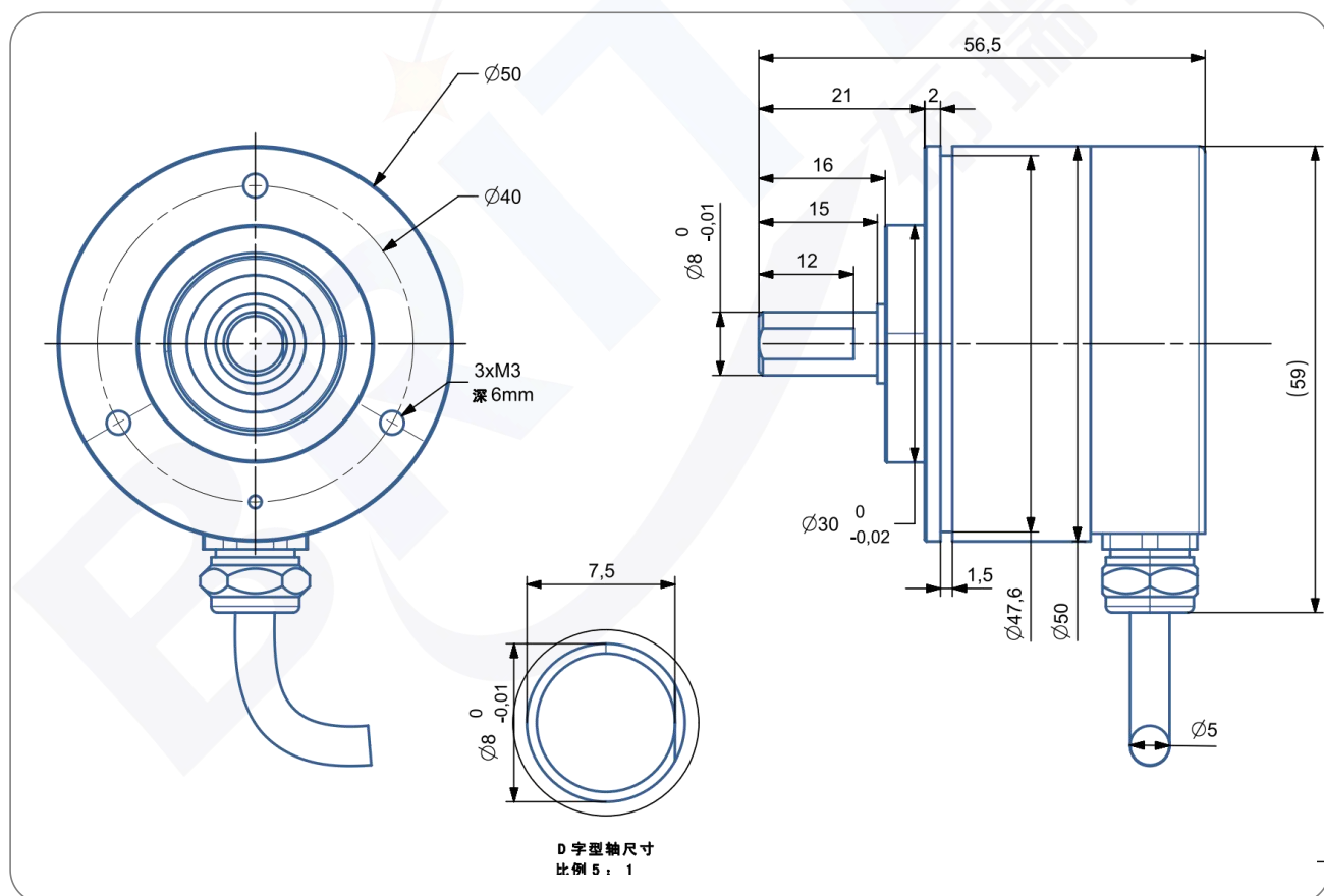
尺寸型号图 10: 输出轴-8mm IP68/防爆
