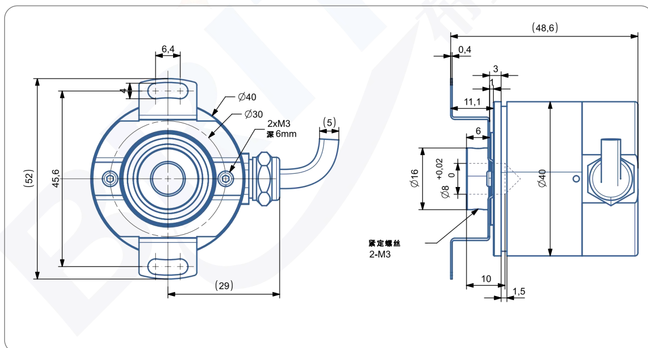
尺寸型号图 8: 输出轴 8mm 盲孔 IP68/防爆
